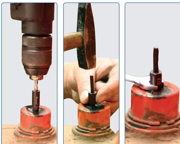
Abb. 1 Abgebrochenes Gewinde mit Bohrhülse anbohren
