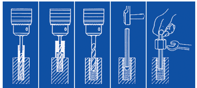
Abb. 1 Abgebrochenes Gewinde mit Bohrhülse anbohren
